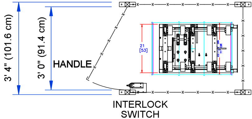
DOOR PANEL
