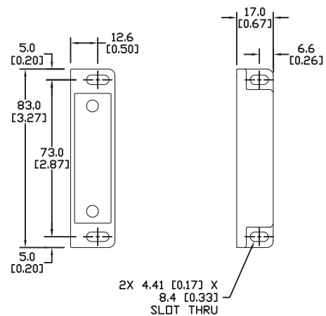
ACTUATOR
